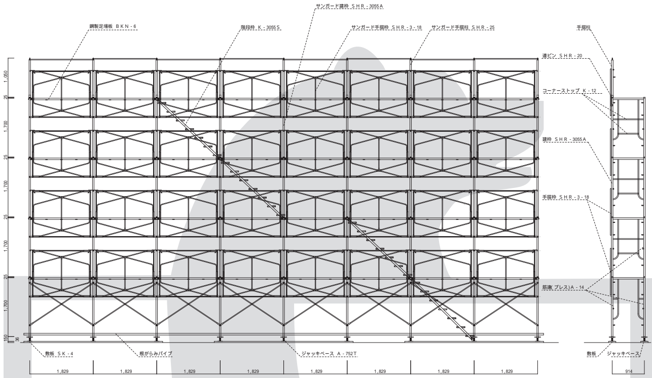
立面図
