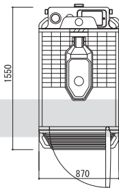
平面図
