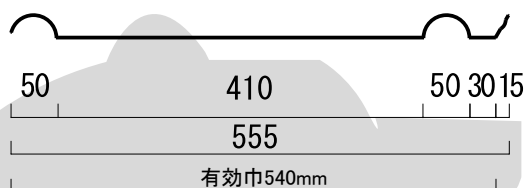
断面図
